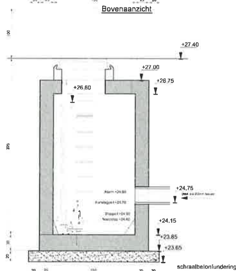
Doorsnede A-A
