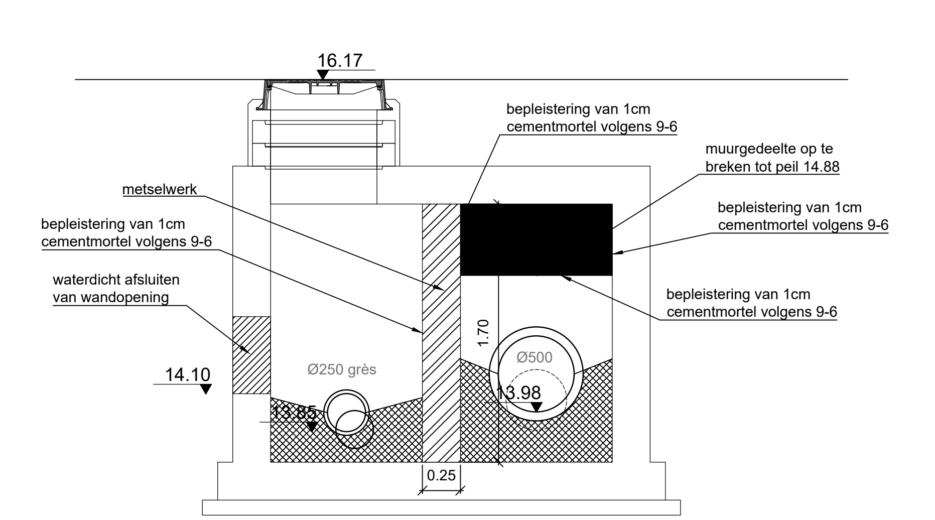
DOORSNEDE A-A'
