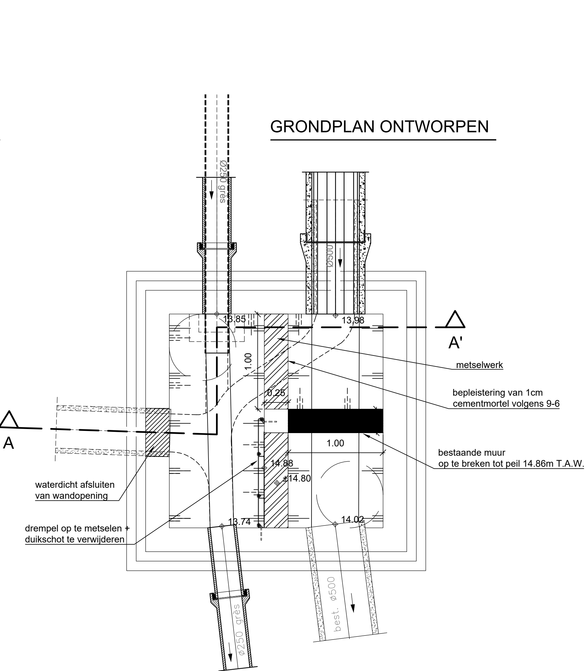
GRONDPLAN BESTAAND
