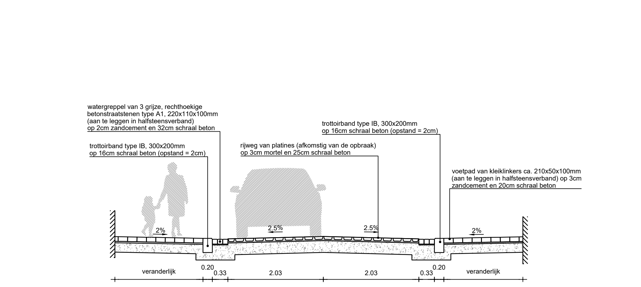
ONTWORPEN SNEDE D-D'
