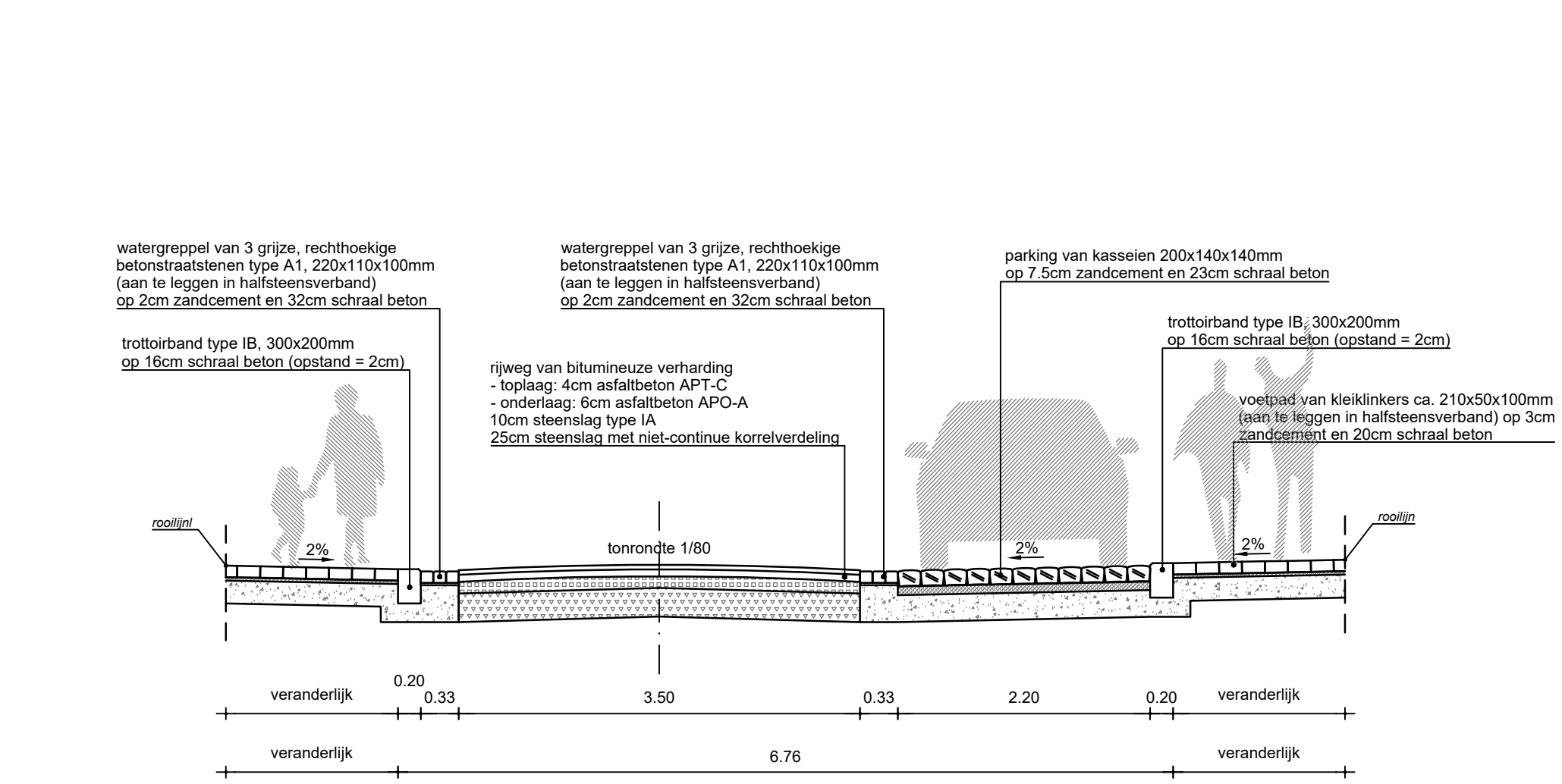
ONTWORPEN SNEDE A-A'
