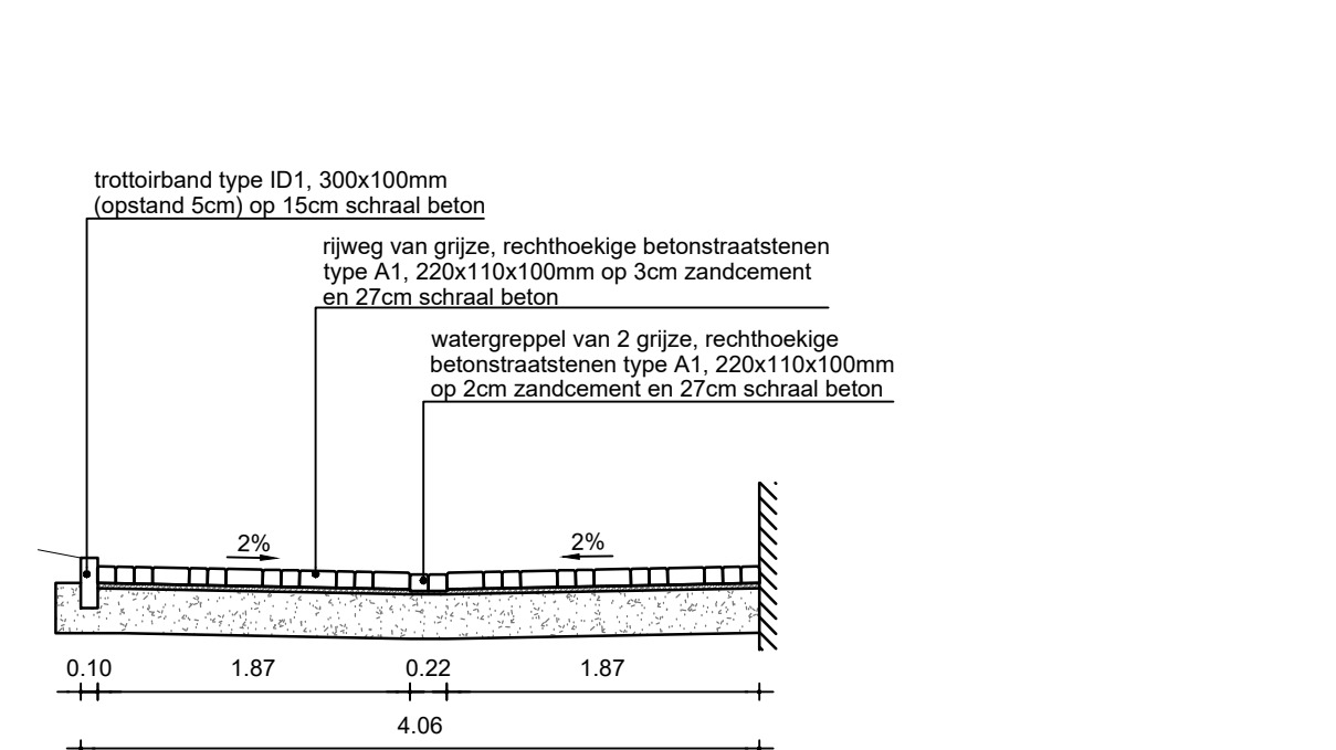
ONTWORPEN SNEDE E-E'
