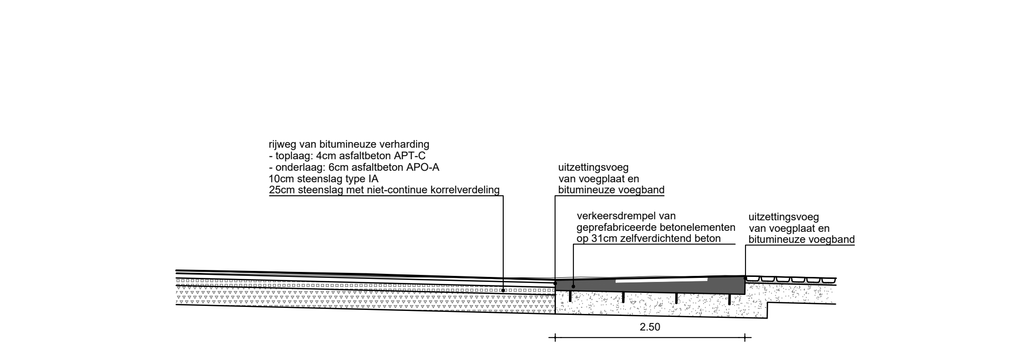
ONTWORPEN SNEDE C-C'
